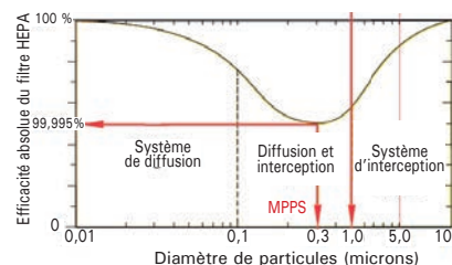
Fig. 1. Efficacité de filtration d'un filtre HEPA. La norme UNE-EN 1822, définit l'efficacité de filtration d'un filtre HEPA comme la performance de filtration de la particule ayant le MPPS (maximum penetration particle size) le plus élevé. Les particules d'environ 0,3 µm sont les plus difficiles à piéger pour un filtre HEPA absolu et c'est ce qui dicte l'efficacité du filtre. Les plus petites nanoparticules sont plus faciles à piéger par diffusion, les plus grosses par impact, inertie et mécanismes d'interception.
