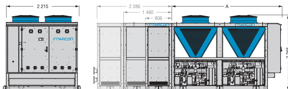
Groupe hydraulique (1)
