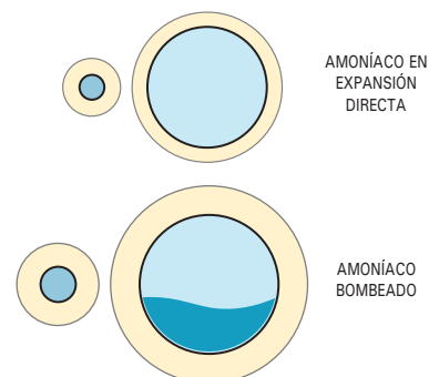
Comparación de tuberías de amoníaco
