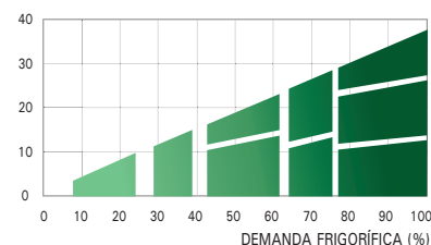
Presión de aspiración en banda neutra
