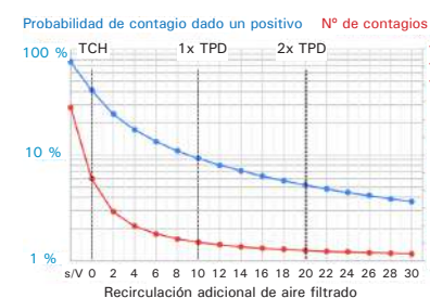
Fig. 2. Simulación de la probabilidad de contagio dado un positivo en una sala de trabajo de 200 m² con 13 trabajadores a una temperatura de 12 °C. Fuente: Prof. José L. Jiménez, Dept. of Chem. and CIRES, Univ. of Colorado-Boulder.
