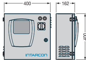
Cotas en mm.
