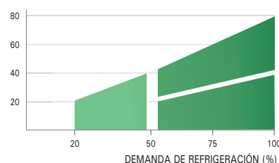
POTENCIA FRIGORÍFICA (kW)
